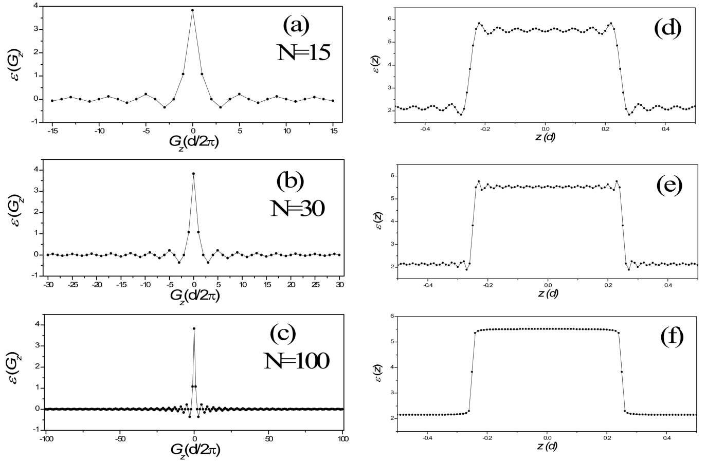
Figura 2. Los paneles (a), (b) y (c) muestran los valores de los coeficientes de Fourier calculados para N=15 , 30 y 100. Los paneles (d), (e) y (f) muestra la función dieléctrica en el espacio real para N=15 , 30 y 100.
